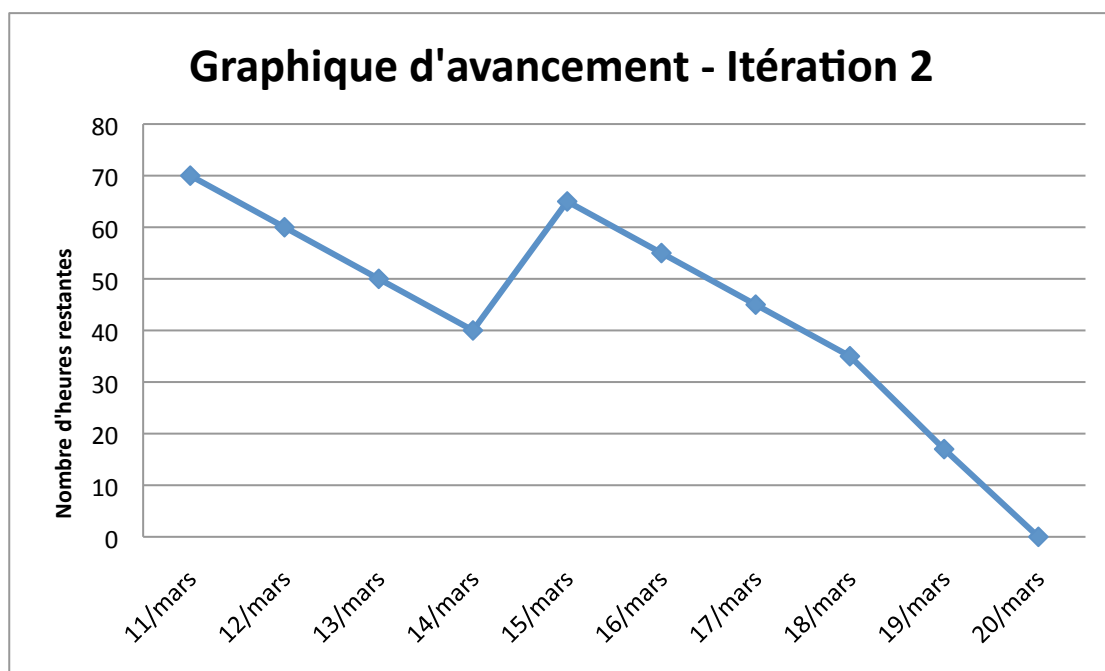
Figure 3 Exemple de graphique d'avancement simple
